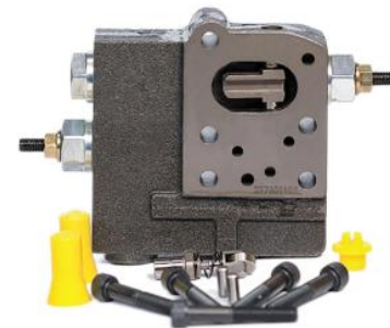
A11VO40/60 LDR
